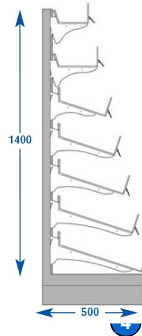
Base Riser
